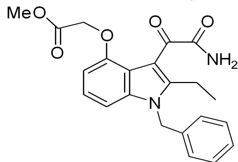
Varespladib Methyl, Lot 02, NMR in CDCL 3
